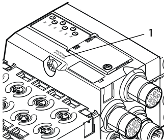
Abb. 12-11 Identifikationsschlüssel des Buskopplers
