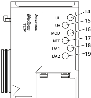
Abb. 10-1 LED-Zustände
