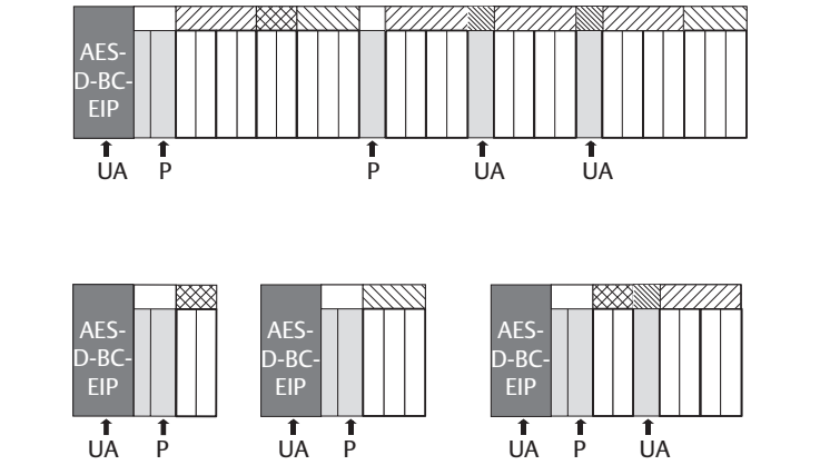
Fig. 12-15 Esempi di configurazioni non consentite
