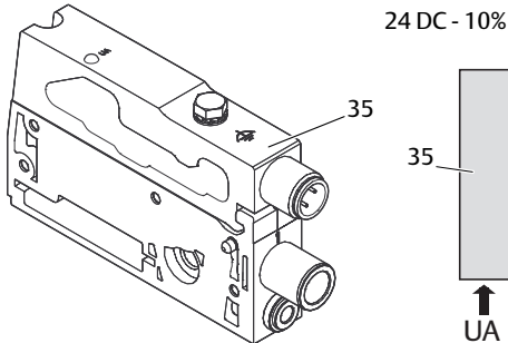
Abb. 12-5 Elektrische Einspeiseplatte
