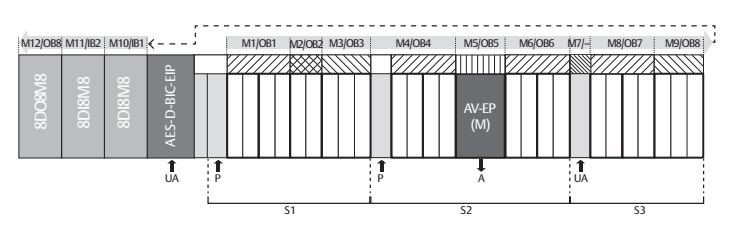
Fig. 5-1 Numeración de los módulos en un sistema de válvulas con módulos E/S
