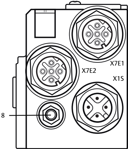
Fig. 4-6 Conexión FE
