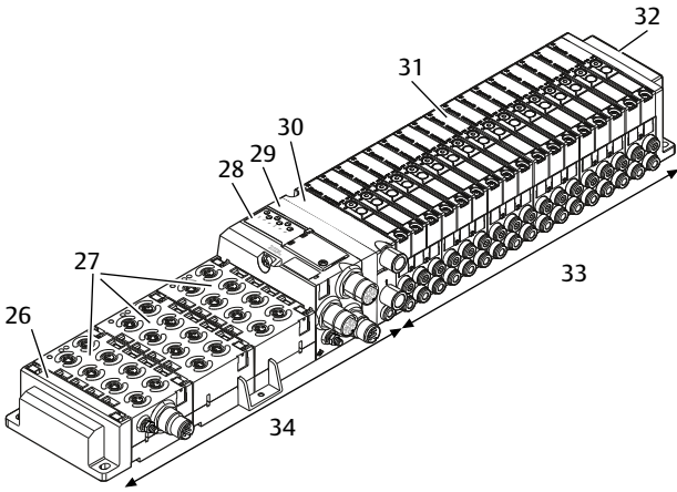
Fig. 12-1 Ejemplo de configuración: unidad formada por acoplador de bus y módulos E/S de la serie AES y válvulas de la serie AV
