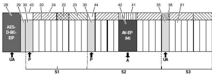
Abb. 12-13 Bildung von Sektionen mit zwei pneumatischen Einspeiseplatten und einer elektrischen Einspeiseplatte
