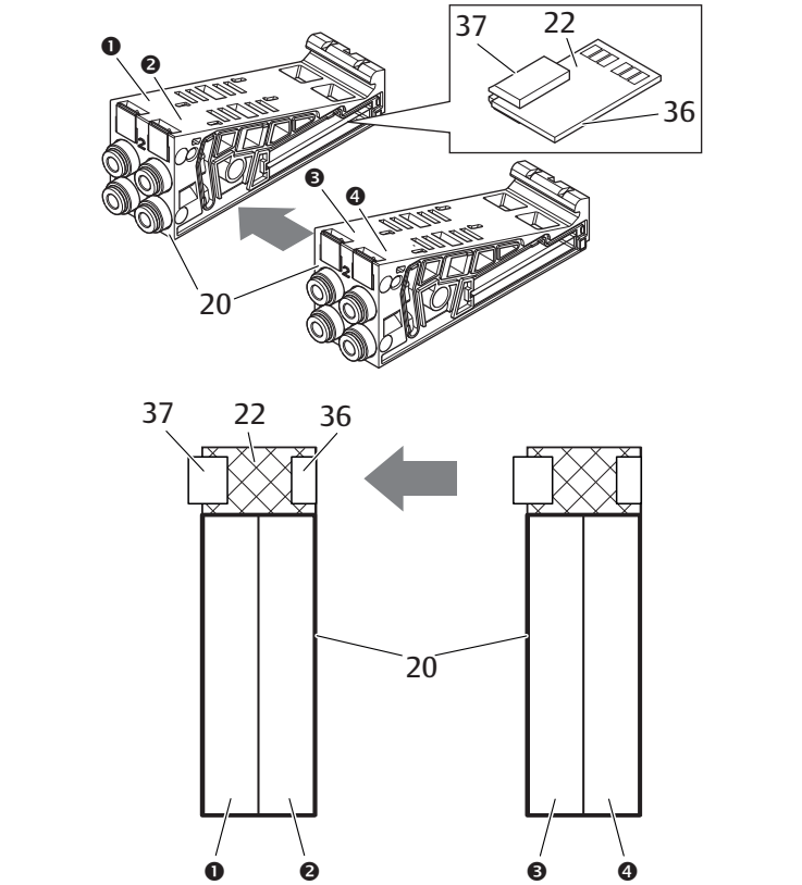
Fig. 12-7 Unión en bloque de placas base y placas de controlador de válvula
