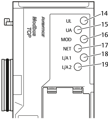
Fig. 4-7 Significado de los LED
