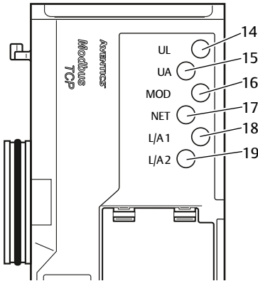
Fig. 10-1 Etats des LED
