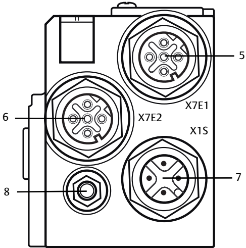
Fig. 4-2 Raccordements électriques du coupleur de bus
