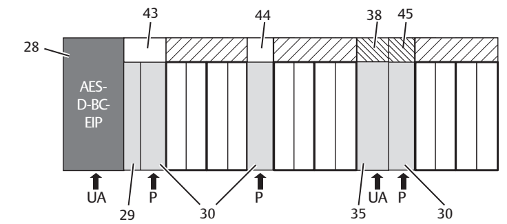
Fig. 12-10 Schede per collegamento a ponte e scheda per collegamento a ponte UA-OFF
