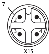
Fig. 4-4 Affectation des broches de l'alimentation électrique
