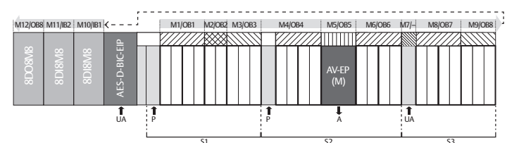
Abb. 5-1 Nummerierung der Module in einem Ventilsystem mit E/A-Modulen
