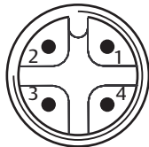
Abb. 12-6 Pinbelegung M12-Stecker
