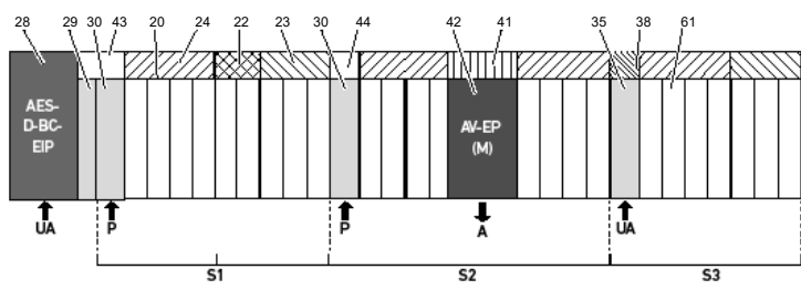
Fig. 12-13 Formación de secciones con dos placas de alimentación neumáticas y una eléctrica
