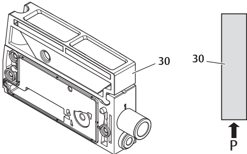
Abb. 12-4 Pneumatische Einspeiseplatte
