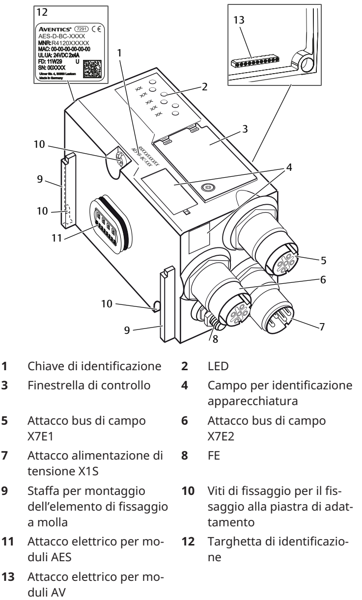
Fig. 4-1 Panoramica sul prodotto accoppiatore bus
