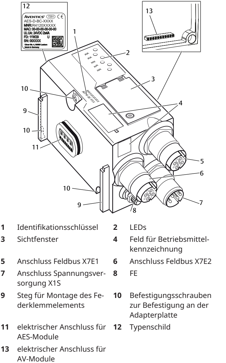
Abb. 4-1 Produktübersicht Buskoppler
