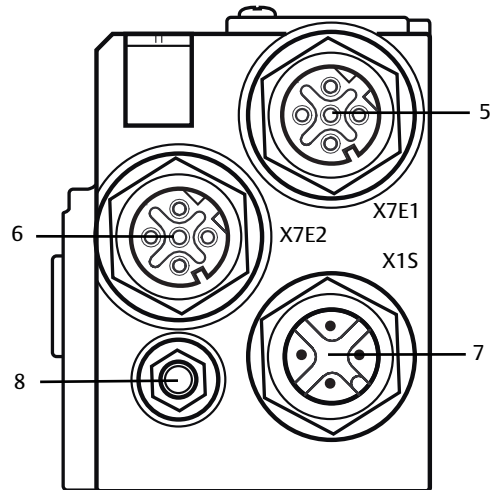
Fig. 4-2 Conexiones eléctricas del acoplador de bus
