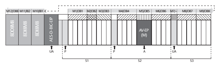
Fig. 5-1 Numérotation des modules dans un îlot de distribution avec modules E/S
