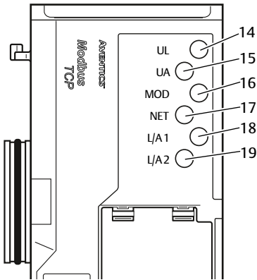
Abb. 4-7 Bedeutung der LEDs
