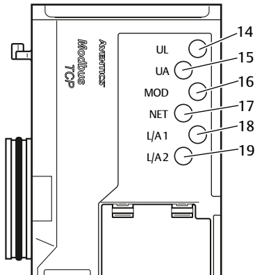
Fig. 11-1 Significado de los LED de diagnóstico
