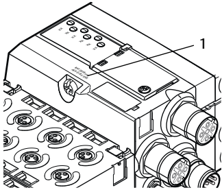
Fig. 12-11 Chiave di identificazione dell'accoppiatore bus
