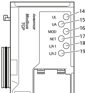
Abb. 11-1 Bedeutung der LED-Diagnose
