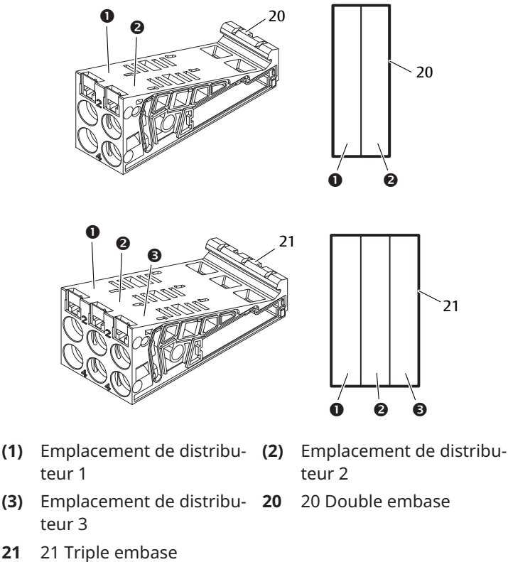
Fig. 12-2 Doubles et triples embases
