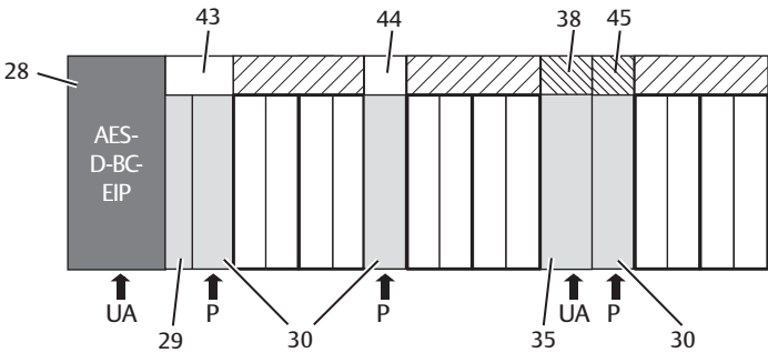
Abb. 12-10 Überbrückungsplatinen und UA-OFF-Überwachungsplatine
