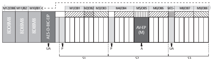
Fig. 5-1 Numerazione dei moduli in un sistema valvole con moduli I/O
