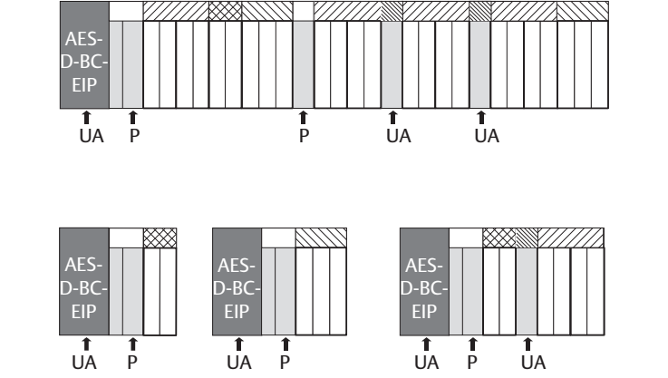
Fig. 12-15 Exemples de configurations non autorisées
