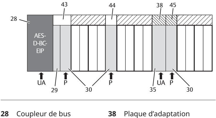
Fig. 12-10 Platines de pontage et platine de surveillance UA-OFF
