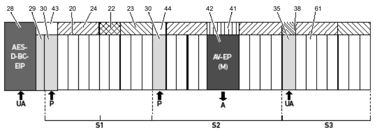
Fig. 12-13 Formation de sections avec deux plaques d'alimentation pneumatiques et une plaque d'alimentation électrique
