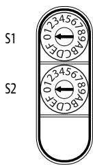
Fig. 4-9 Commutateurs rotatifs S1 et S2
