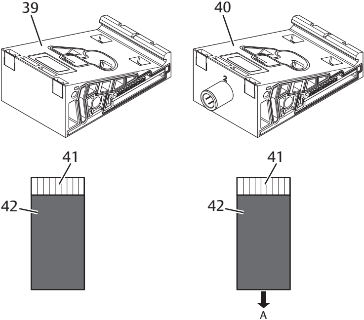
Fig. 12-9 Placas base para válvulas reguladoras de presión para regulación de zona de presión (izquierda) y para regulación de presión única (derecha)
