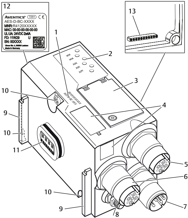
Fig. 4-1 Vue d'ensemble du coupleur de bus
