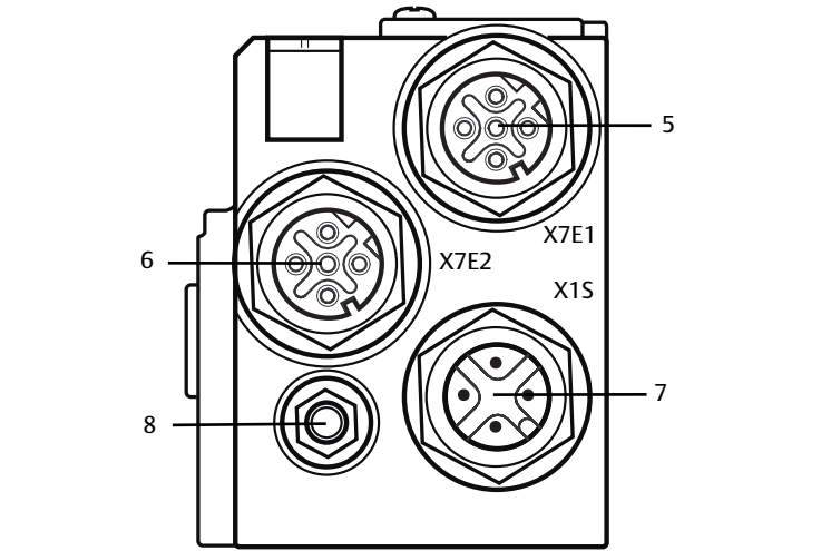
Fig. 4-2 Connessioni elettriche dell'accoppiatore bus
