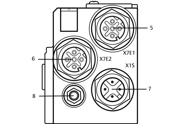
Abb. 4-2 Elektrische Anschlüsse des Buskopplers
