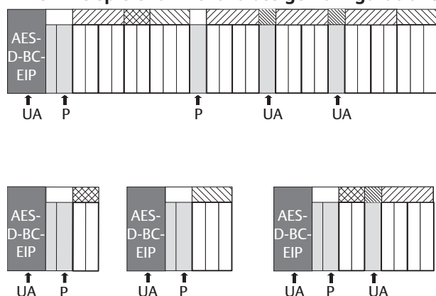
Abb. 12-15 Beispiele für nicht zulässige Konfigurationen
