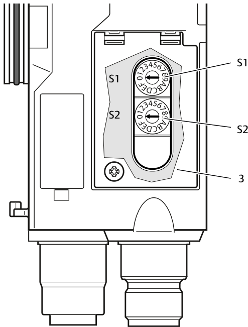
Fig. 4-8 Position des commutateurs d'adresse S1 et S2
