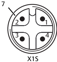
Fig. 4-4 Ocupación de pines Alimentación de tensión
