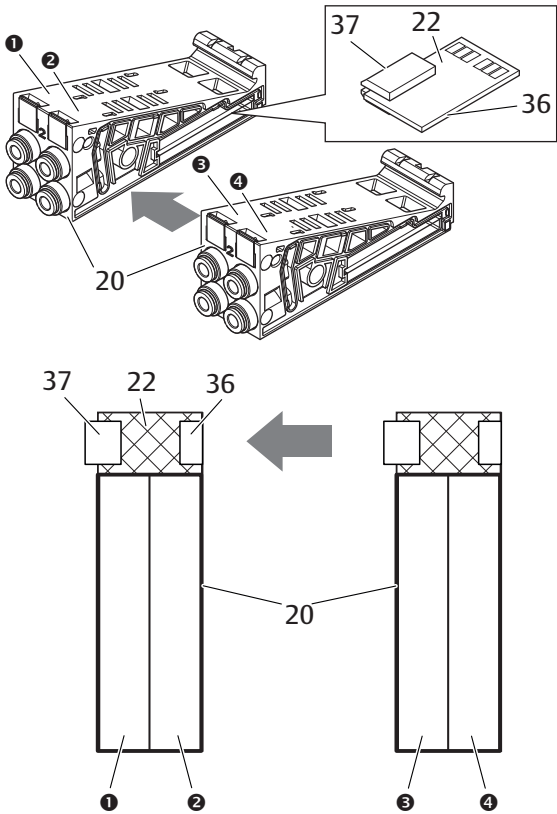
Abb. 12-7 Verblockung von Grundplatten und Ventiltreiberplattenen
