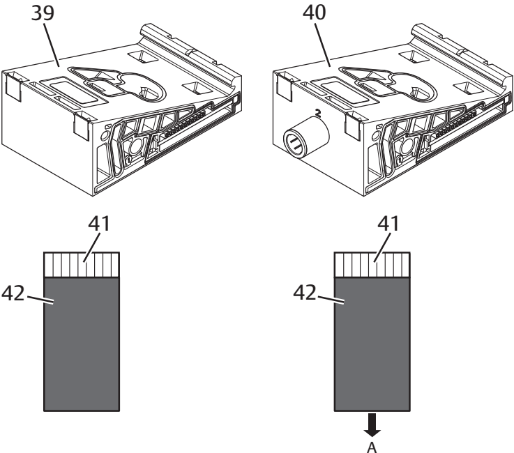
Abb. 12-9 Grundplatten für Druckregelventile zur Druckzonenregelung (links) und Einzeldruckregelung (rechts)
