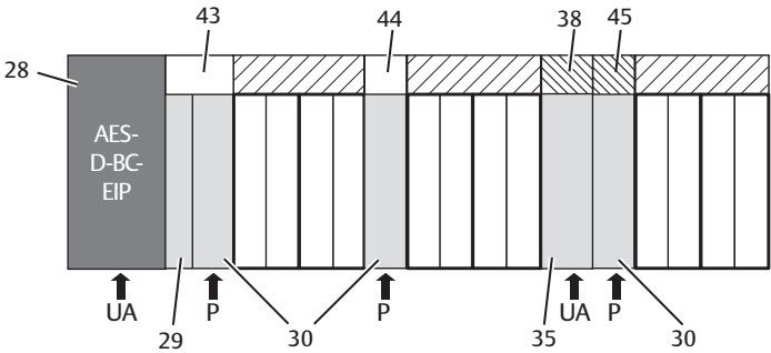
Fig. 12-10 Placas de puenteo y placa de supervisión UA-OFF
