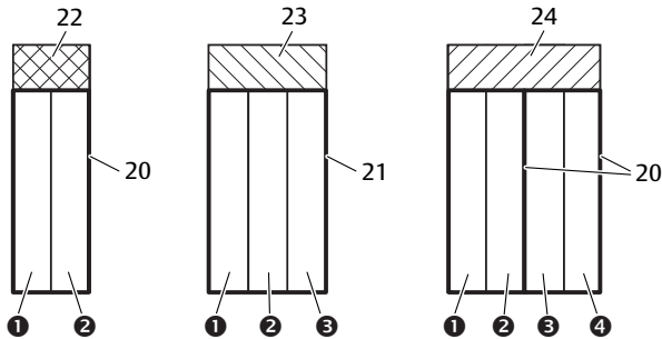
Fig. 6-1 Assegnazione dei posti valvola
