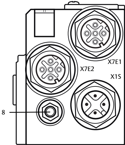
Abb. 4-6 FE-Anschluss
