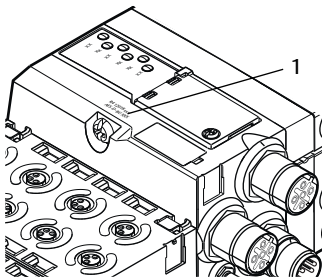
Fig. 12-11 Código de identificación del acoplador de bus
