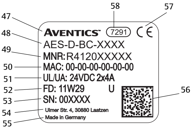
Abb. 12-12 Typenschild des Buskopplers
