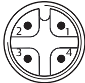
Fig. 12-6 Affectation des broches connecteur M12
