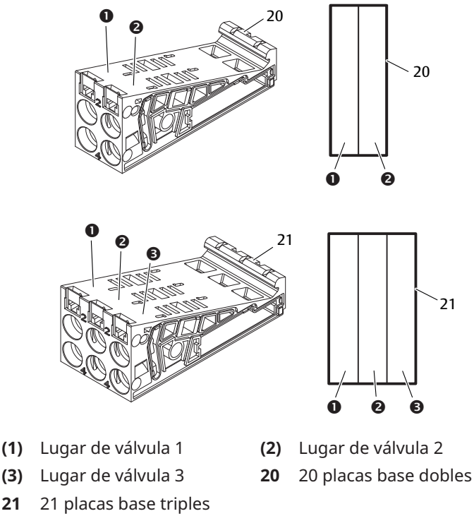
Fig. 12-2 Placas base dobles y triples
