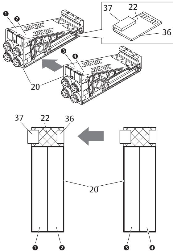
Fig. 12-7 Montaggio in batteria delle piastre base e delle schede driver valvole
