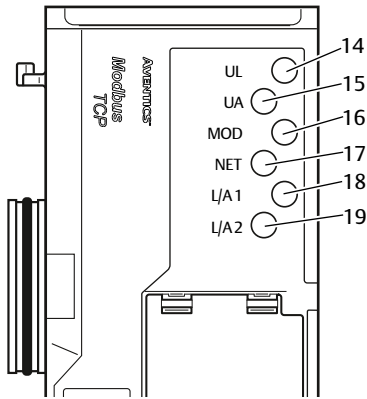
Fig. 11-1 Signification du diagnostic par LED
