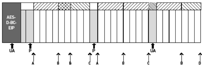
Fig. 12-14 Configuraciones admisibles
