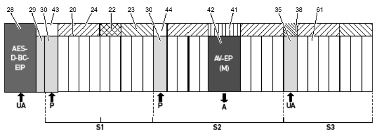
Fig. 12-13 Formazione di sezioni con due piastre di alimentazione pneumatica e una piastra di alimentazione elettrica
