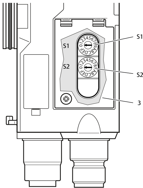
Fig. 4-8 Posición de los conmutadores de dirección S1 y S2
