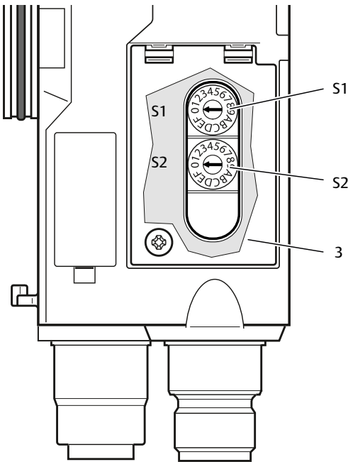
Fig. 4-8 Posizione dei selettori indirizzo S1 e S2
