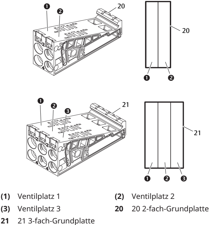
Abb. 12-2 2-fach- und 3-fach-Grundplatten
