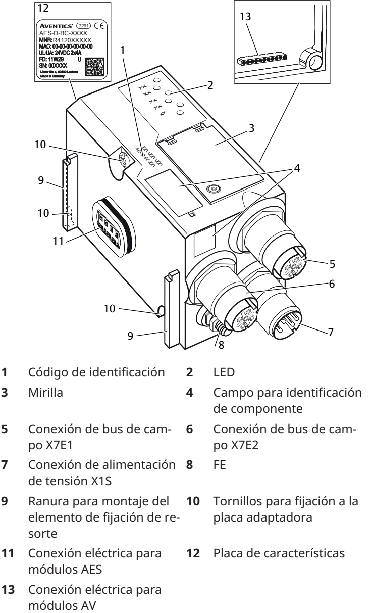
Fig. 4-1 Vista general de productos Acopladores de bus
