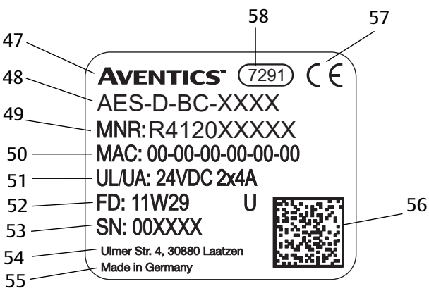
Fig. 12-12 Placa de características del acoplador de bus
