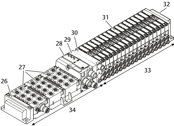
Fig. 12-1 Esempio di configurazione: unità composta da accoppiatore bus e moduli I/O della serie AES e valvole della serie AV
