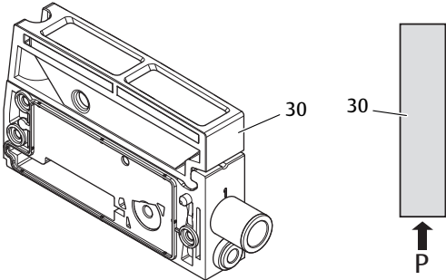
Fig. 12-4 Placa de alimentación neumática
