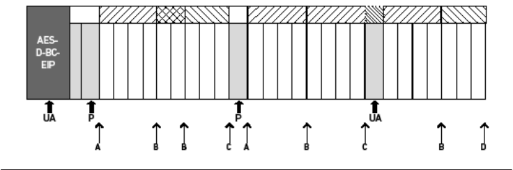
Abb. 12-14 Zulässige Konfigurationen
